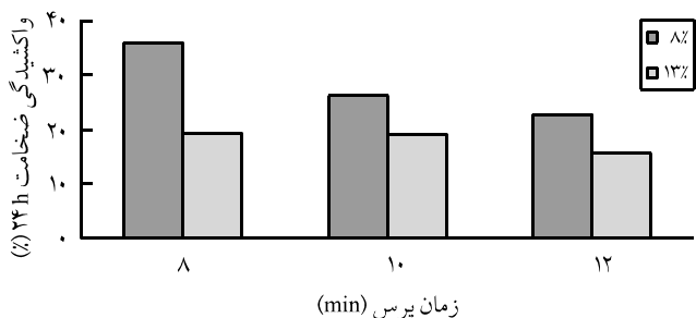
شکل ۱۴ - مقایسه بین واکشیدگی ضخامت 24 h تخته‌های ساخته شده از رزین AESO.
