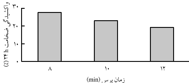
شکل ۱۳ - اثر مستقل زمان پرس بر واکشیدگی ضخامت 24 h تخته‌های ساخته شده از رزین AESO.
