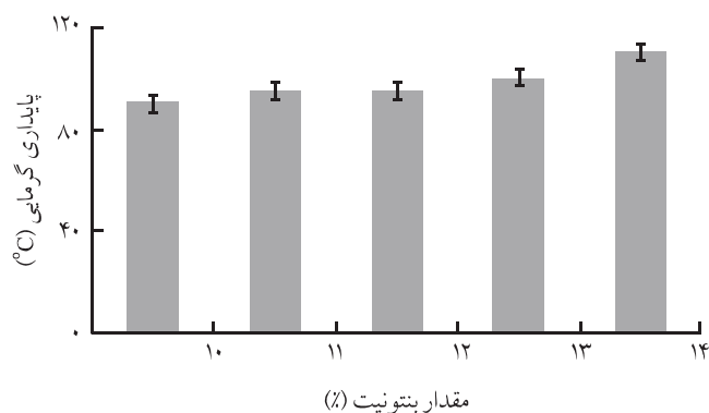
شکل ۳- اثر مقدار بنتونیت روی پایداری گرمایی امولسیون.
