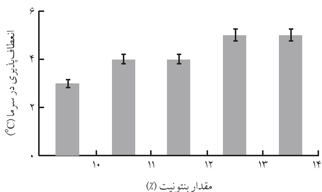
شکل ۴- اثر مقدار بنتونیت روی مقاومت انعطاف‌پذیری در سرمای امولسیون.
