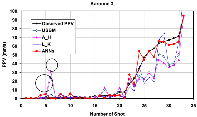
شکل ۷- ب: نمودار گرافیکی مقایسه بین مقدار ثبت شده شدت لرزش و تخمین مدل‌های مختلف برای ساختگاه کارون ۳.
