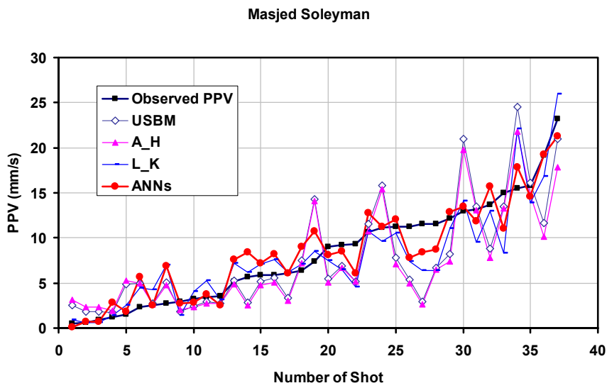
شکل ۶: نمودار گرافیکی مقایسه بین مقدار ثبت شده شدت لرزش و تخمین مدل‌های مختلف برای ساختمان مسجد سلیمان.
