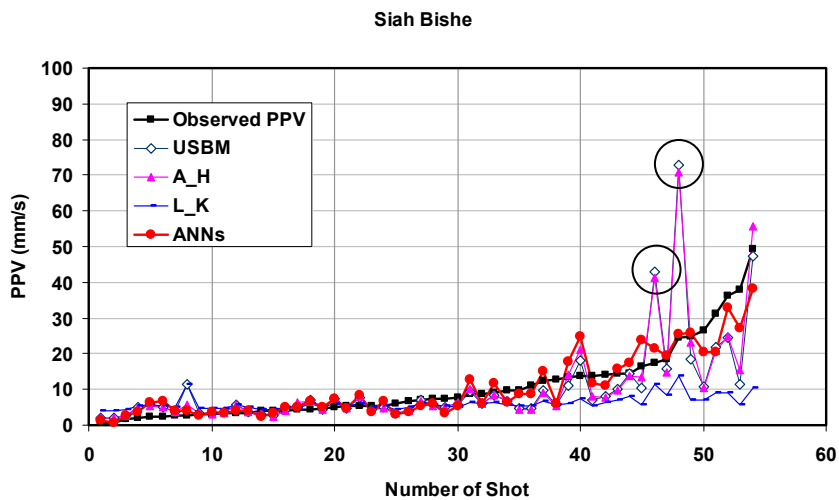
شکل ۸- ب: نمودار گرافیکی مقایسه بین مقدار ثبت شده شدت لرزش و تخمین مدل‌های مختلف برای ساختگاه سیاه بیشه.
