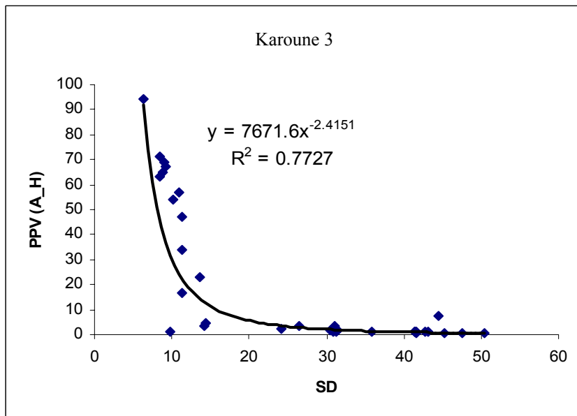
شکل ۷- الف: منحنی رگرسیونی PPV در مقابل فاصله مقیاس شده برای ساختمان کارون ۳.
