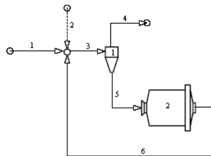
شکل ۶: فلوشیت مدار شبه‌سازی شده توسط نرم‌افزار BMCS.
