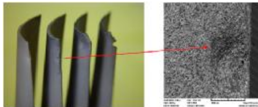
شکل ۱: تصویر خسارت دیده چند نمونه از پره توربین گاز موتور جت در اثر FOD.
