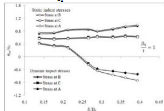
شکل ۲۵: مقایسه بین تنش‌های پسماند شبه استاتیکی و دینامیکی بر حسب \frac{\delta}{D_2}
