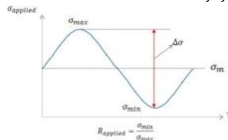
شکل ۶: نمودار بار اعمالی به جسم مکعبی شکل.
