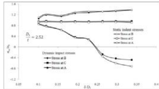
شکل ۲۳: مقایسه بین تنش‌های پسماند شبه استاتیکی و دینامیکی بر حسب \frac{\delta}{D_2}
