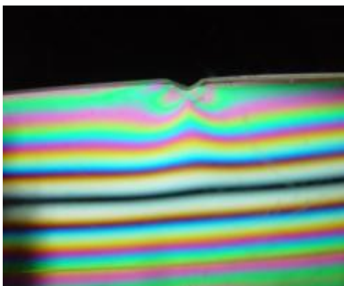
شکل ۱۵: آنالیز تجربی تنش برای فرورفتگی با \frac{\delta}{D_1} = 0.09375 و w = 1.86 \text{ mm} را نشان می‌دهد که ضریب تمرکز تنش را برای بستر حفره به دست می‌دهد. K_T = \frac{\sigma}{\sigma_0}
