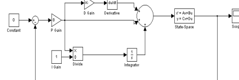
شکل ۲۲: بلوک دیاگرام مدار بسته کنترل موقعیت میکرو زبردربایی.
