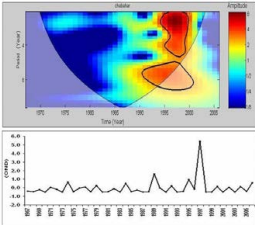
شکل ۵: تحلیل طیفی موجک پیوسته و سری زمانی استاندارد شده بارش فصل پاییز چابهار
