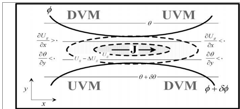
شکل ۲) گردش عمودی در منطقه ورودی و خروجی یک رودباد راست‌خست. UVM و DVM به ترتیب نماینده حرکات عمودی صعودی و نزولی هستند (مارتین، ۲۰۰۶، برگردان از: مسعودیان، ۱۳۸۸: ۲۶۹).
