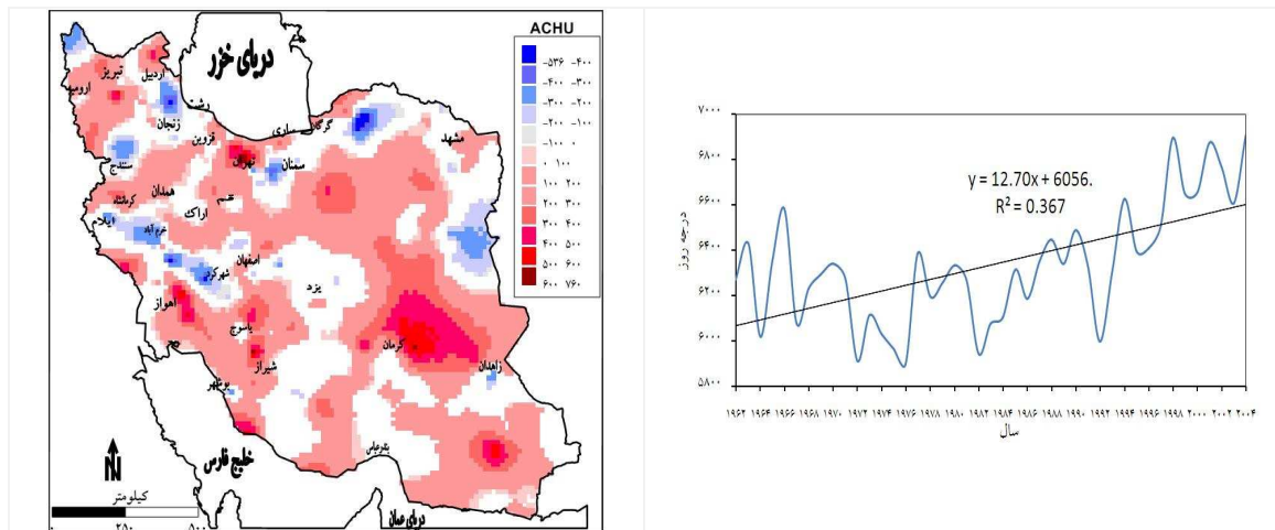
نگاره ۷) پراکنش مکانی مناطق دارای روند و شیب روند شاخص واحد گرمای محصول (ACHU) بر حسب مقدار در دهه (چپ) و روند شاخص برای کل ایران بر حسب مقدار در سال (راست)
