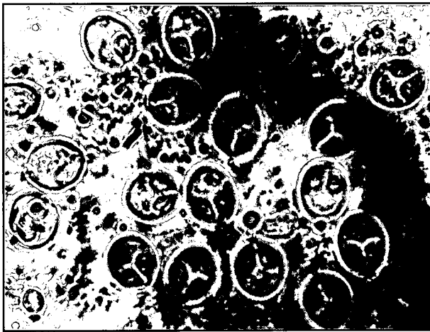
تصویر ۲- اسپور انگل میکسوبولوس کوالی جدا شده از کیست شعاعهای ثانویه آبشش ماهی B. mursa بدون رنگ آمیزی، بزرگنمایی ۱۷۵۰.
