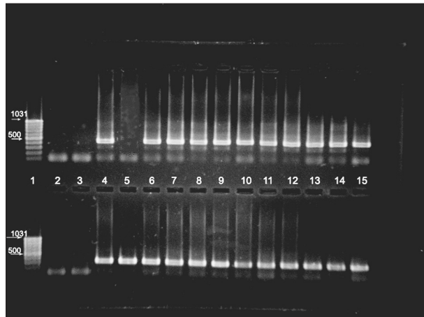
تصویر ۱- محصولات ۴۳۴bp حاصل از آزمون PCR، پس از استفاده از آغازگر شناساگر ردیف ۱۳۲bp تکرار شونده (ردیف بالا)، محصولات ۳۱۴bp پس از استفاده از آغازگر شناساگر ژن آنتی ژن A (ردیف پایین) ستون ۱: مارکر ۱۰۰bp، ستون ۲: بلانک، ستون ۳: کنترل منفی (DNA لکوسیت های یک مرغ فاقد علائم)، ستون ۴: تومور عضله سینه، ستون ۵: واکسن دوگانه HVT-Rispens، ستون ۶، ۷ و ۸: طحال، ستون ۹، ۱۰ و ۱۱: کبد، ستون ۱۲: تخمدان، ستون ۱۳: پیش معده، ستون ۱۴ و ۱۵: بورس فابریسیوس.
