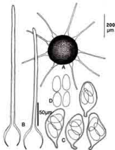
شکل ۸- Phyllactinia sp. روی Salix aegyptiaca (A) آسکوکارپ، (B) زواید درفشی، (C) آسک‌های حاوی ۳ آسکوسپور، (D) آسکوسپورها. Fig. 8. Phyllactinia . sp. ex Salix aegyptiaca : A. Ascocarp, B. acicular appendages, C. asci with 3 ascospores, D. ascospores.
