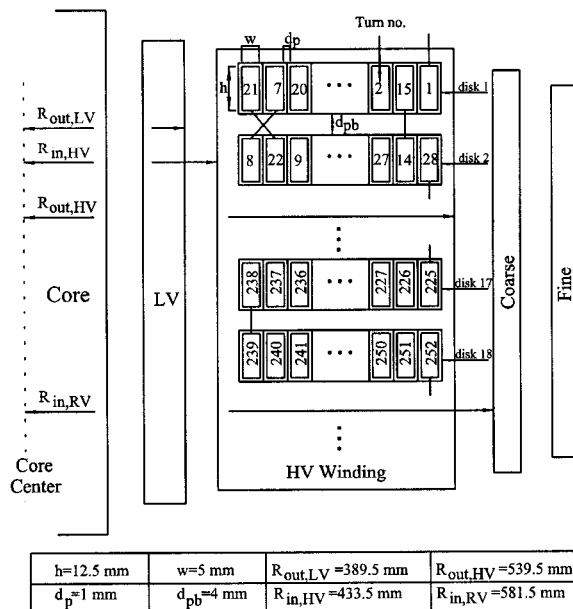
شکل (3): ساختار ترانسفورماتور 132kV/20kV
