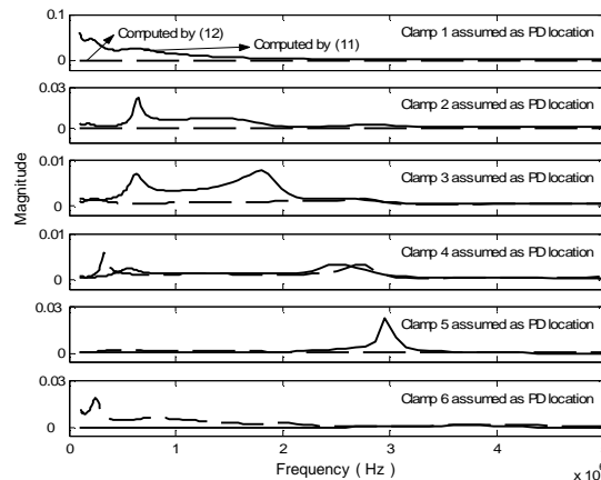
شکل (16): دو سیگنال محاسبه شده بوسیله (11) و (12) و تئیکه PD
