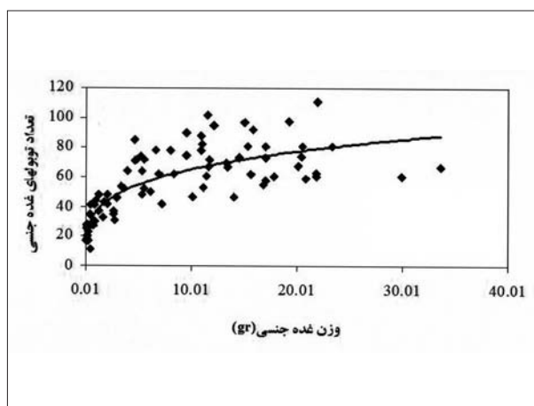
تصویر ۴- نمودار ارتباط بین تعداد توبول‌های غده جنسی و وزن غده جنسی نر (بیضه). R^2=0.7379, y=37.045x^{0.2467}
