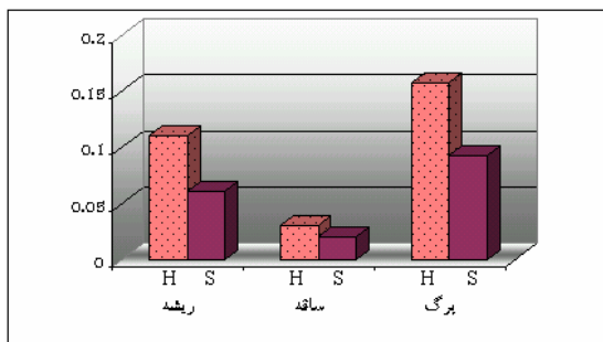
شکل ۴- مقایسه میزان آلکالوئیدهای هیوسیامین و اسکوپولامین در اندامهای مختلف گیاه H. pusillus در مرحلهٔ رویشی در منطقهٔ
