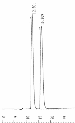
شکل ۲- کروماتوگرام حاصل از HPLC محلول استاندارد اسکوپولامین (1) و هیوسیامین (2)
