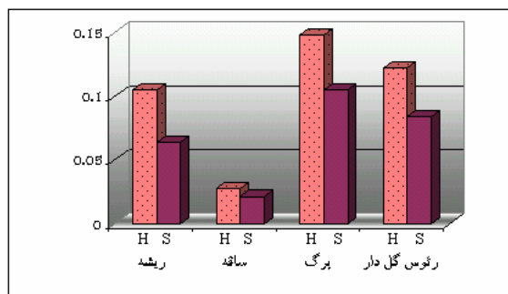
شکل ۷- مقایسه میزان آلکالوئیدهای هیوسیامین و اسکوپولامین
