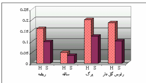
شکل ۶ - مقایسه میزان آلکالوئیدهای هیوسیامین و اسکوپولامین
