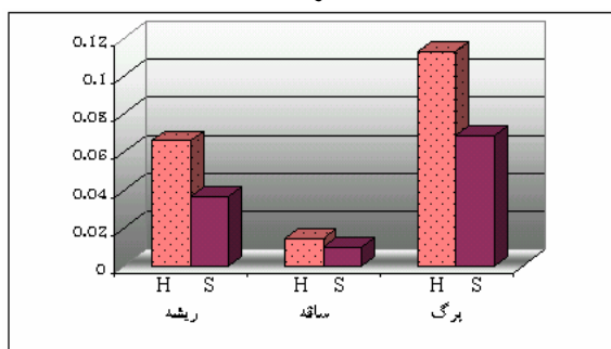
شکل ۵- مقایسه میزان آلکالوئیدهای هیوسیامین و اسکوپولامین در اندامهای مختلف گیاه H. pusillus در مرحلهٔ رویشی در منطقهٔ
