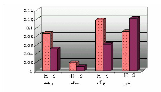
شکل ۹- مقایسه میزان آلکالوئیدهای هیوسیامین و اسکوپولامین
