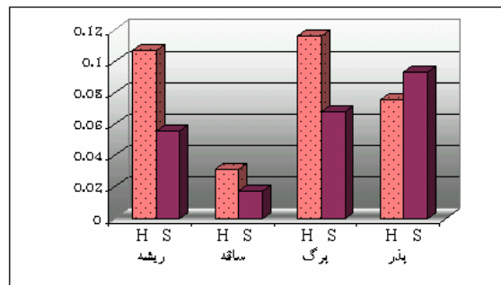
شکل ۸- مقایسه میزان آلکالوئیدهای هیوسیامین و اسکوپولامین
