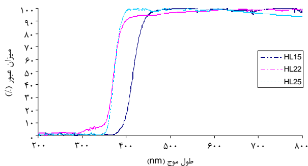
HL, hydrophilic intraocular lens نمودار ۲- طیف عبور نور از لنزهای هیدروفیل
