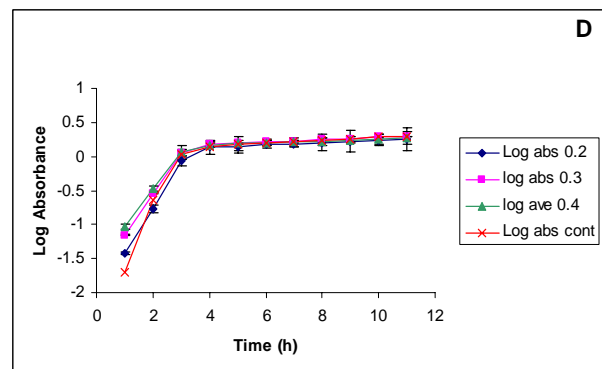
شکل ۱: منحنی رشد باکتری 0157 E. coli تحت تاثیر غلظت‌های مختلف ۰/۲ (A)، ۰/۳ (B)، ۰/۴ (C) میلی لیتر عصاره الکلی گیاه اوکالیپتوس Eucalyptus globulus مقایسه اثر غلظت‌های مختلف بر رشد باکتری در مقایسه با کنترل در نمودار D نشان داده شده است.
