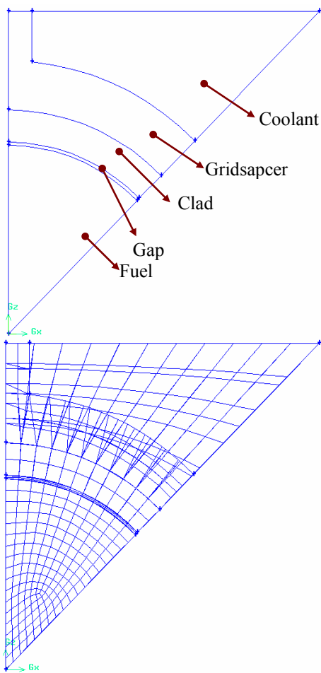
شکل ۱۳- نحوه مدل‌سازی و شبکه‌بندی یک هشتم میله
