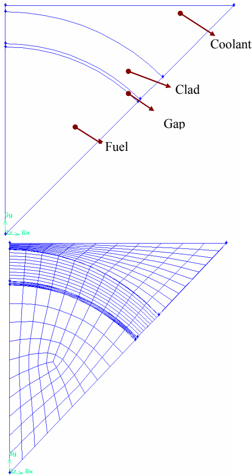
شکل ۳- نحوه مدل سازی و شبکه بندی یک هشتم میله
