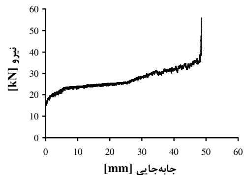
شکل ۱۵- منحنی نیرو- جابه‌جایی آزمایشگاهی برای لوله سه کنگره‌ای در قالب باز
