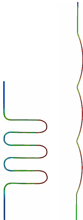
شکل ۱۱- بارگذاری محوری بیش از حد و چروکیدگی ناشی از آن، بدست آمده از شبیه‌سازی برای لوله مسی شکل یافته در قالب بسته سه کنگره‌ای
