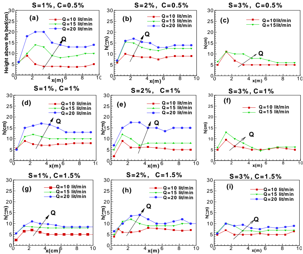
شکل ۳- ارتفاع جریان گل آلود در طول کانال و نسبت به تغییرات دبی، شیب و غلظت
