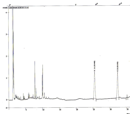
شکل ۱: کروماتوگرام استاندارد اسید اروسیک و استاندارد داخلی (هنیکوزانوییک اسید)
