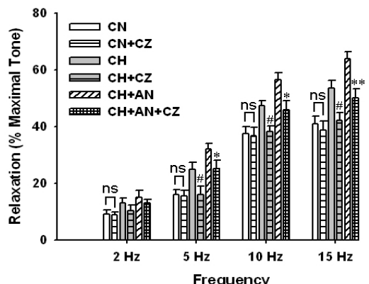
شکل - ۳: کاپسازین در گروه sham (CN+CZ) هیچ اثری بر پاسخ‌های شل‌شدگی به تحریک الکتریکی در بافت کورپوس کاورنوزوم نداشت، ولی موجب جلوگیری از افزایش این پاسخ‌ها در گروه سروتیک (CH+AN) شد. ( p < 0.05 ، p < 0.01 و p < 0.001 در مقایسه با گروه سروتیک در حضور آنانداماید؛ # p < 0.05 در مقایسه با گروه سروتیک بدون آنانداماید؛ ns به معنای غیر معنی‌دار)
