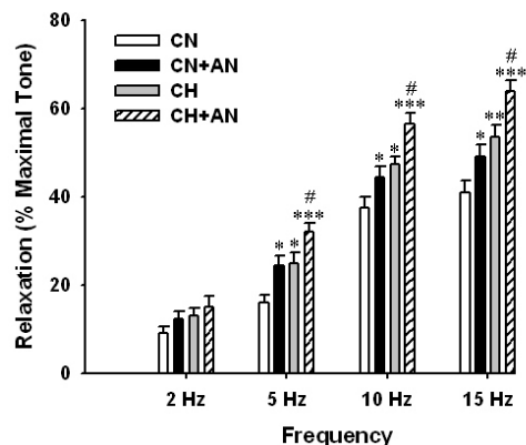
شکل - ۱: پاسخ‌های شل‌شدگی به تحریک الکتریکی در بافت کورپوس کاورنوزوم در گروه‌های (sham (CN)، سروتیک (CH)، sham در حضور آنانداماید (CN+AN) و سروتیک در حضور آنانداماید (CH+AN)، p < 0.05 در مقایسه با گروه سروتیک بدون آنانداماید. p < 0.01 و p < 0.001 در مقایسه با گروه sham بدون آنانداماید؛ # p < 0.05 در مقایسه با گروه سروتیک بدون آنانداماید.
