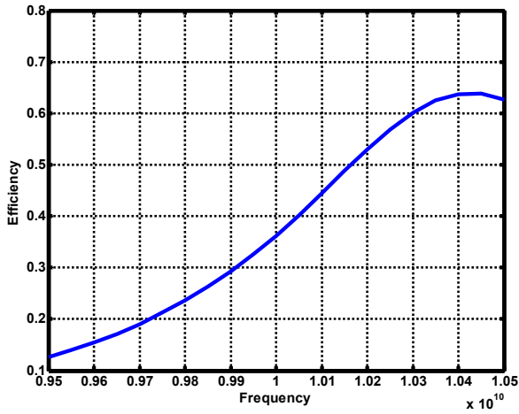
شکل ۱۷: بازدهی نسبت به فرکانس برای تغییر فازی به اندازه 30^\circ .
