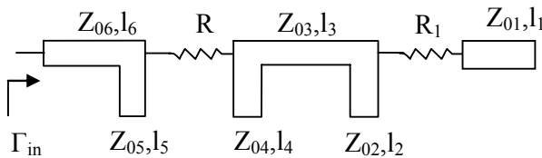
شکل ۷: ساختار مدار تغییر دهنده فاز با تلفات پیشنهادی.
