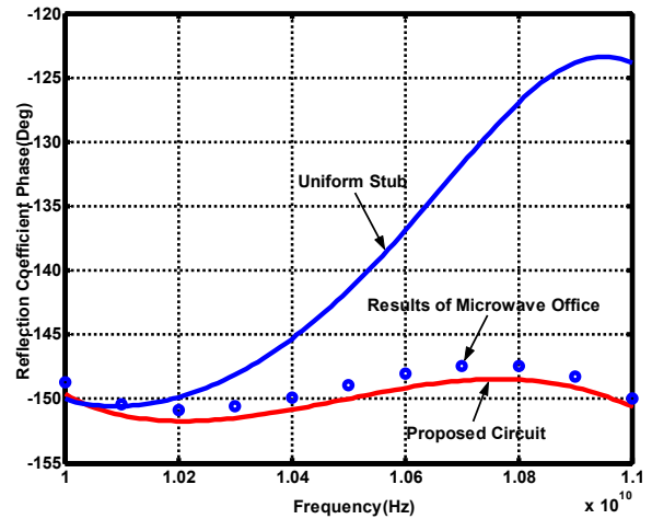
شکل ۱۶: پاسخ فاز ضریب انعکاس مدار تغییر دهنده فاز راکتیو برای تغییر فاز 150^\circ .
