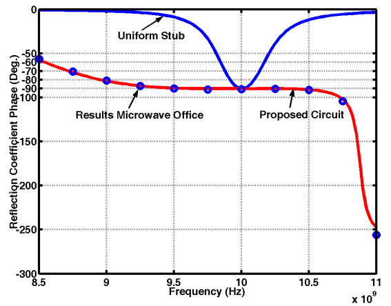
شکل ۱۲: پاسخ فاز ضریب انعکاس برای تغییر فاز معین -90^\circ در مورد تغییر دهنده فاز با تلفات و شاخک یکنواخت.
