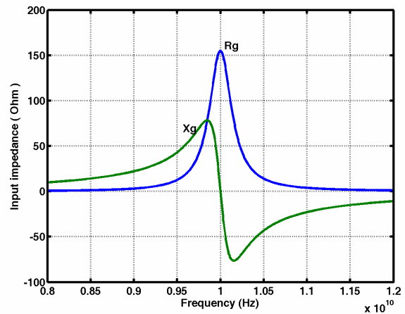
شکل ۴: تغییرات فرکانسی امپدانس ورودی یک پچ مستطیلی با مشخصات h = 0.381 mm و \varepsilon_r = 2.33 ، L = 9.24 mm، W = 13.84 mm 10 GHz
