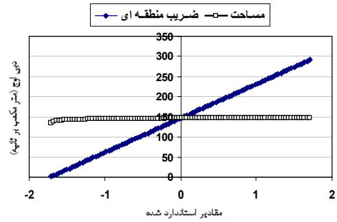
شکل ۶. نمودار آنالیز حساسیت متغیرهای رابطه کریگر
