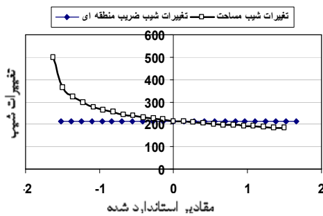
شکل ۷. تغییرات شیب متغیرهای رابطه دیکن
