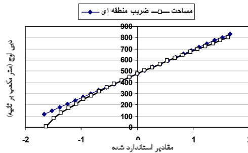
شکل ۸. نمودار آنالیز حساسیت متغیرهای رابطه دیکن
