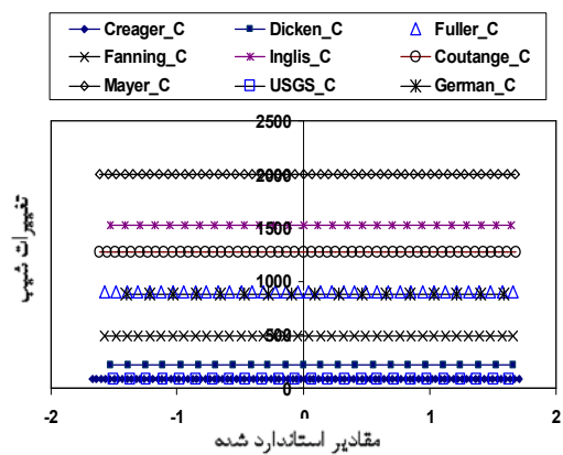
شکل ۹. حساسیت روابط مختلف نسبت به تغییرات ضریب منطقه‌ای
