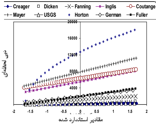
شکل ۱۱. مقایسه حساسیت ده رابطه مذکور در مقابل متغیرهای آنها
