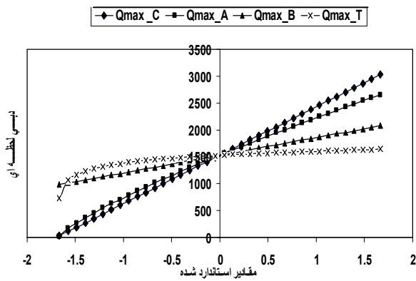
شکل ۱۲. نمودار آنالیز حساسیت پارامترهای رابطه فولر
