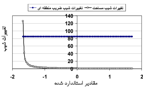
شکل ۵. تغییرات شیب متغیرهای رابطه کریگر
