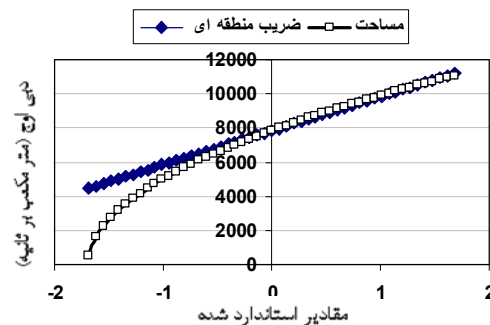
شکل ۱۲. نمودار آنالیز حساسیت متغیرهای رابطه مایر
