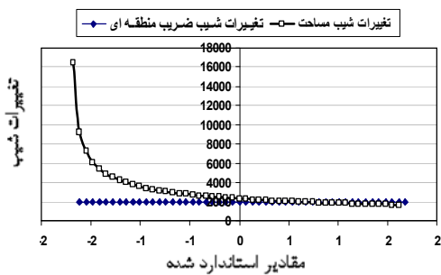
شکل ۱۱. تغییرات شیب متغیرهای رابطه مایر
