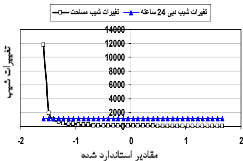
شکل ۹. تغییرات شیب متغیرهای رابطه فولر
