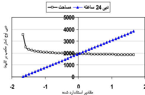
شکل ۱۰. نمودار آنالیز حساسیت متغیرهای رابطه فولر
