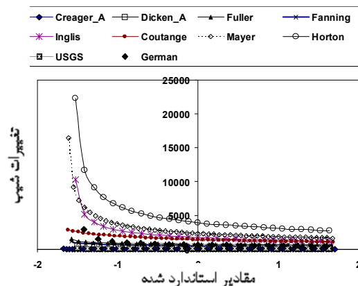
شکل ۱۰. حساسیت روابط مختلف نسبت به تغییرات فاکتور مساحت
