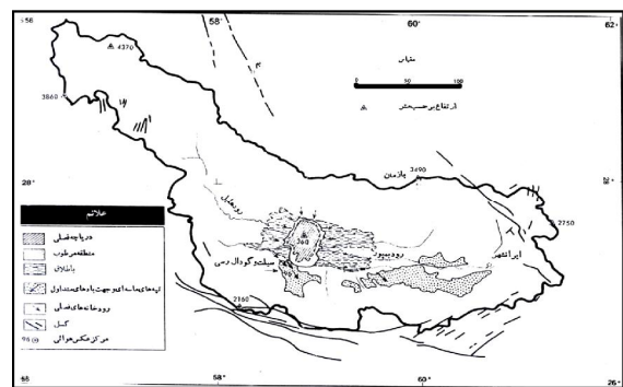
شکل ۱. فرونشست جازموریان و پلایای فصلی هامون جازموریان
