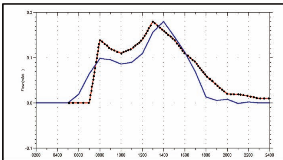
شکل ۵: هیدروگراف مشاهده‌ای و محاسباتی مدل بعد از واسنجی برای سیلاب ۷۳/۰۹/۱۰
