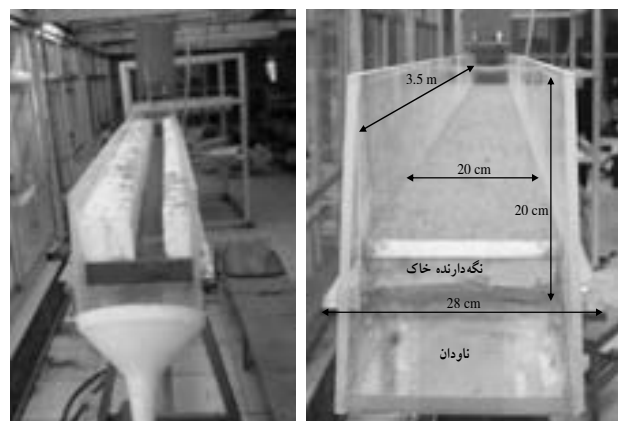
شکل ۱. کانال و بستر فرسایشی مورد استفاده
