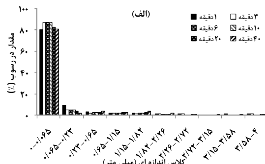
شکل ۴. تغییرات توزیع اندازه ذرات رسوب در نمونه خاک گیلوان در قدرت جریان‌های الف (۰٫۱۲، ب) ۰٫۲، ج) ۰٫۳، د) ۰٫۴، ه) ۰٫۶، و و) ۰٫۸ وات بر متر مربع
