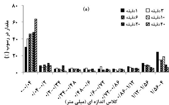
شکل ۴. تغییرات توزیع اندازه ذرات رسوب در نمونه خاک گیلوان در قدرت جریان‌های الف (۰٫۱۲، ب) ۰٫۲، ج) ۰٫۳، د) ۰٫۴، ه) ۰٫۶، و و) ۰٫۸ وات بر متر مربع
