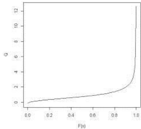
شکل (۵): منحنی چندک‌های برآورد شده توزیع منطقه‌ای GLO برگزیده برای منطقه‌ی همگن اول.
