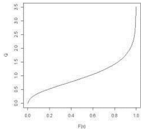
شکل (۶): منحنی چندک‌های برآورد شده توزیع منطقه‌ای PE3 برگزیده برای منطقه‌ی همگن دوم.
