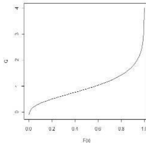
شکل (۱): منحنی چندک‌های برآورد شده توزیع منطقه‌ای GNO برگزیده برای منطقه‌ی همگن.
