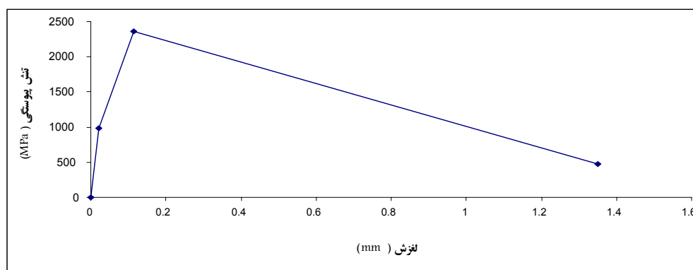
شکل ۵: نمودار تنش پیوستگی-نغزش برای فنر غیر خطی.
