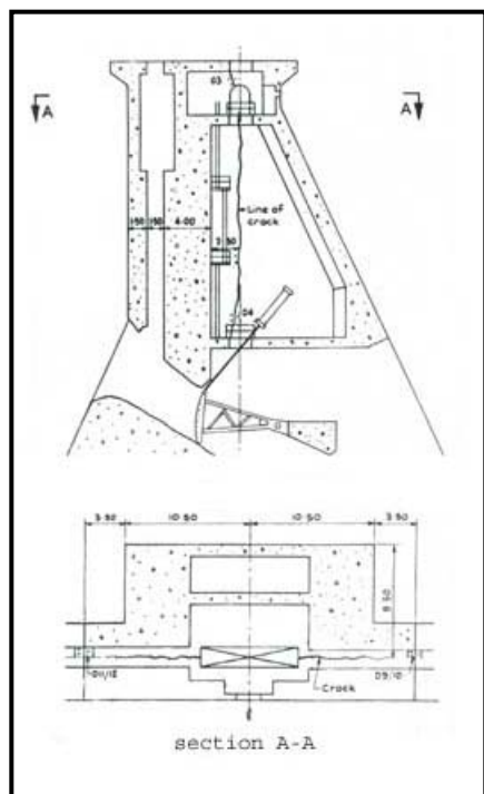
شکل ۱: موقعیت و امتداد ترک در بلوک ۱۰/۱۱.
