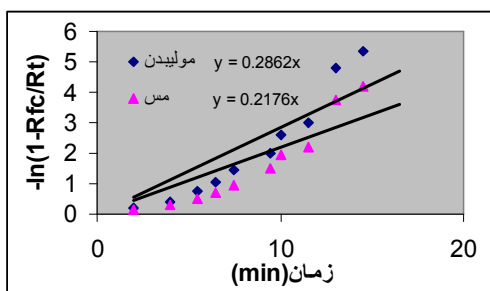
شکل ۲: نمودار تعیین ثابت سینتیکی برای مس و مولیبدن در آزمایش S-12.
