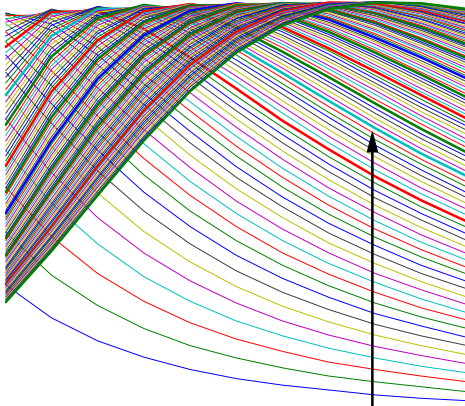
شکل ۳: تغییرات حاصلضرب کارائی سرریزوروشن شدگی روزنه برحسب فاصله کانونی برای مقادیر مختلف n(1,2,\dots,120) .
