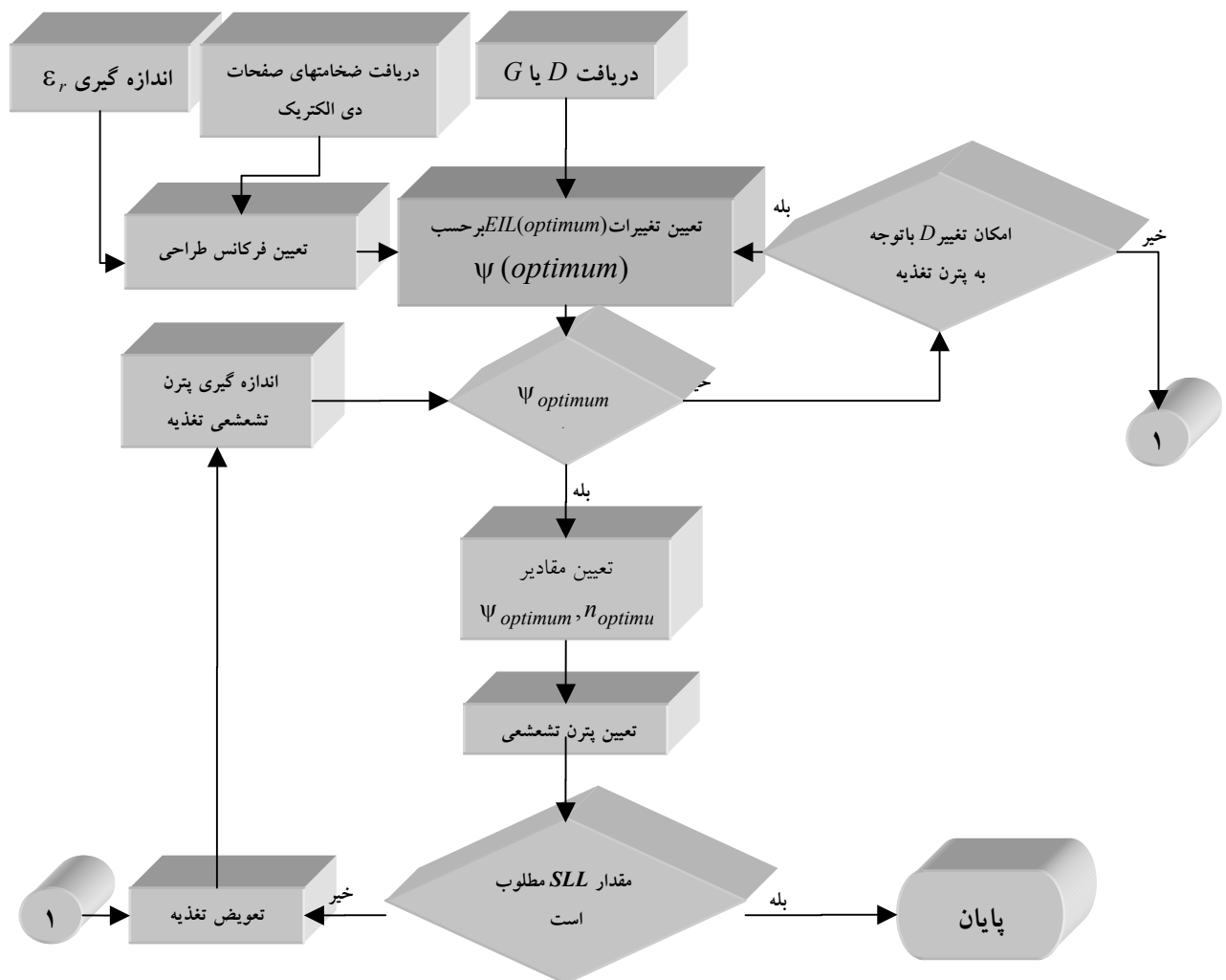
شکل ۱۴: فلوجارت مراحل طراحی .
