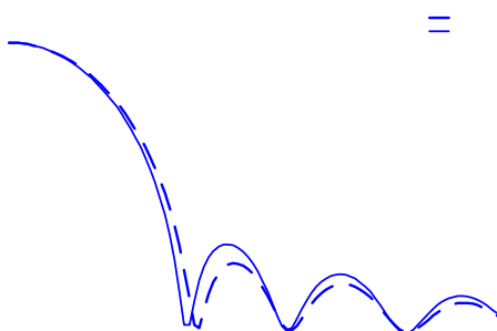
شکل ۱۱: پترن تشعشعی آنتن برای \phi = 0 ، \phi = \pi/2
