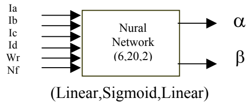
شکل ۸: ساختار شبکه عصبی بکار رفته برای تخمین \alpha, \beta .
