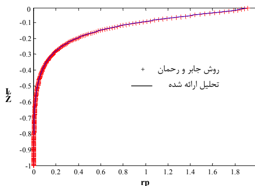
شکل ۵: نمودار نسبت فشار منفذی بی‌بعد در عمق (مقایسه نتایج روش رحمان و جابر با تحلیل ارائه شده).
