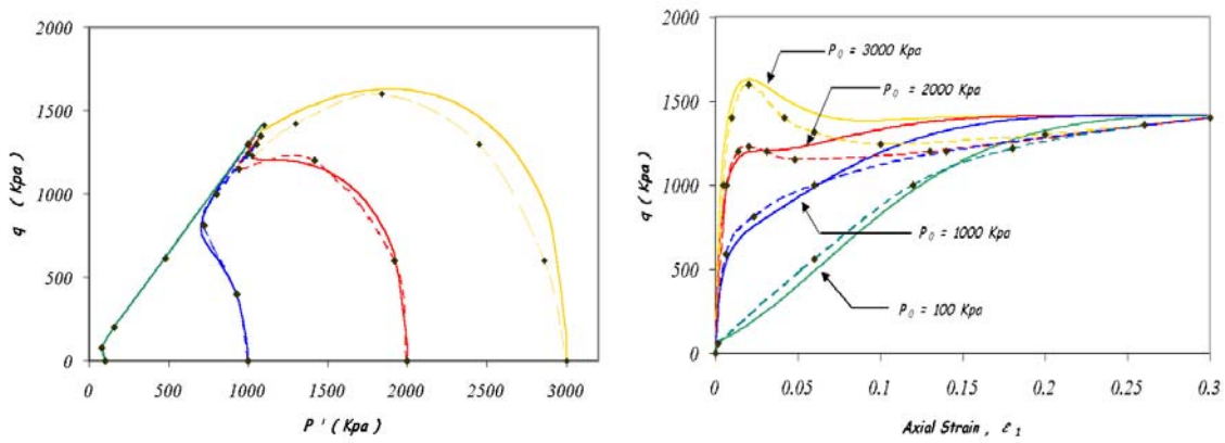
شکل ۶: مقایسه بین نتایج پیش بینی مدل اصلاح شده با داده های تجربی مرجع [ ۱۵ ] برای ماسه توپورا ( e = 0.833 ) در بارگذاری زهکشی نشده.
