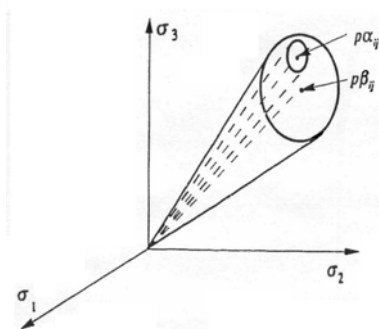
شکل ۲: جایجایی سطح تسلیم در فضای تنشها.
