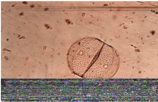
شکل ۴: Hemiaulus
