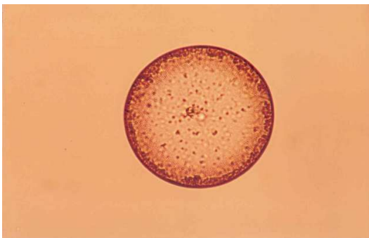
شکل ۶: Stephanodiscus
