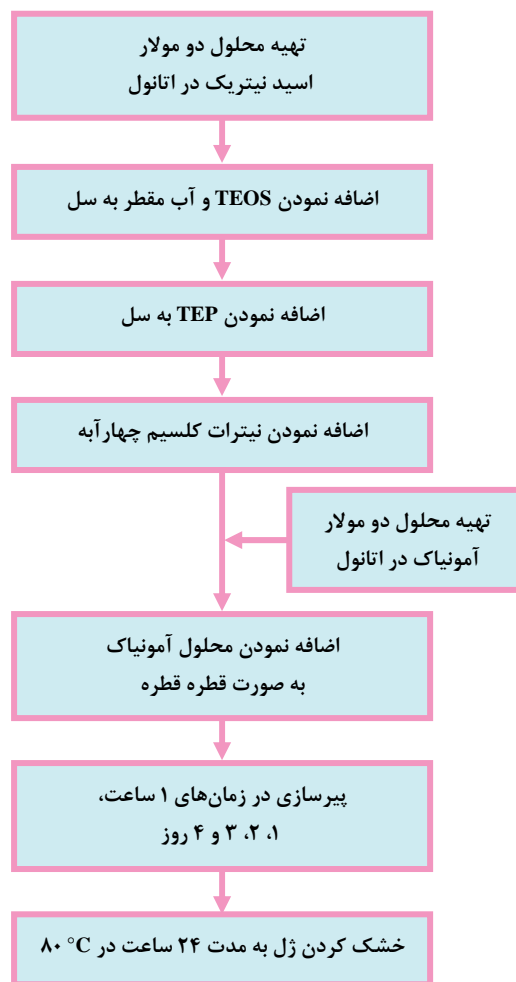
شکل ۱: دیاگرام تهیه نانوپودر شیشه زیستی با استفاده از روش سل-ژل.
