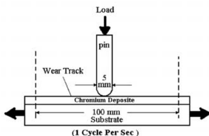
شکل ۱- شماتیک آزمایش سایش رفت و برگشتی
