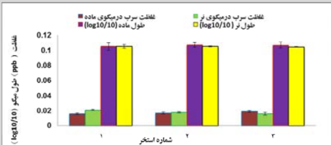
نمودار 2- مقایسه تجمع سرب در میگو با طول میگو در استخرهای شماره 1 تا 3 مرحله دوم سایت حله
