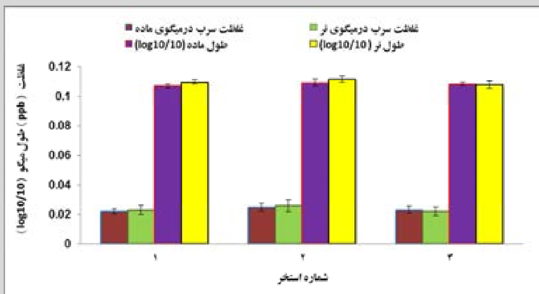
نمودار 3- مقایسه تجمع سرب در میگو با طول میگو در استخرهای شماره 1 تا 3 در حله سوم سایت حله
