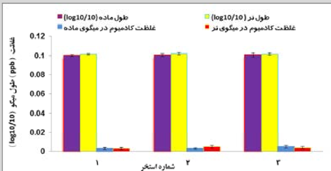
نمودار 4- نمودار مقایسه تجمع کادمیوم در میگو با طول میگو در استخرهای شماره 1 تا 3 در حله اول سایت حله
