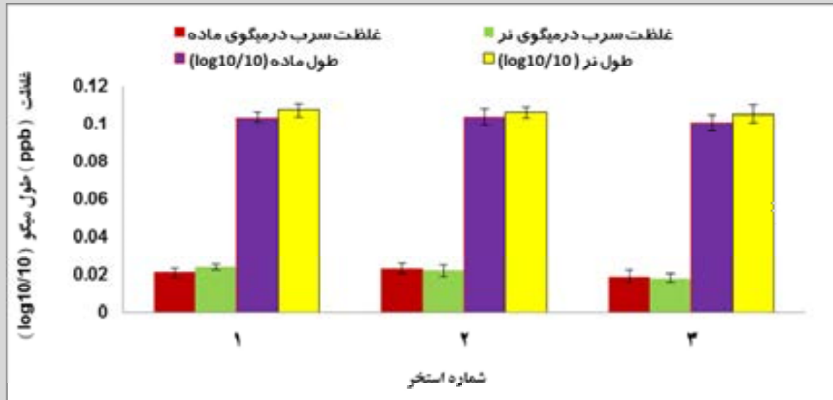
نمودار 7- مقایسه غلظت سرب در میگو با طول میگو در استخرهای شماره 1 تا 3 مرحله اول سایت شیف
