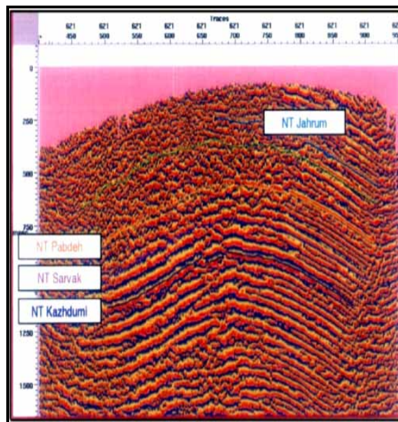
شکل ۵: نشانگر فاز لحظه‌ای بر روی خط امتدادی ۶۲۱
