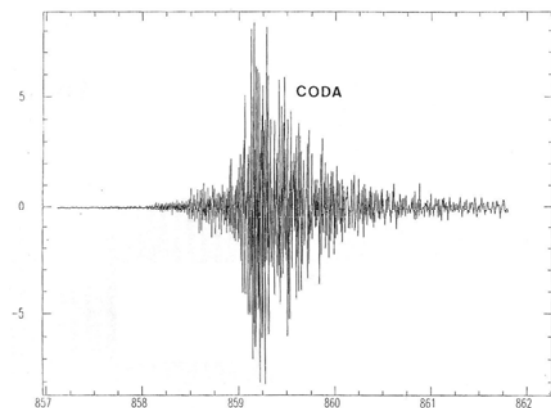
شکل ۲- لرزه نگاشت یک زلزله نزدیک که در آن امواج coda نشان داده شده است. (ایستگاه SFUCBB، زلزله ۲۱ می ۱۹۹۷، \Delta = 324 km (آدپاس آ. ۱۹۹۹))
