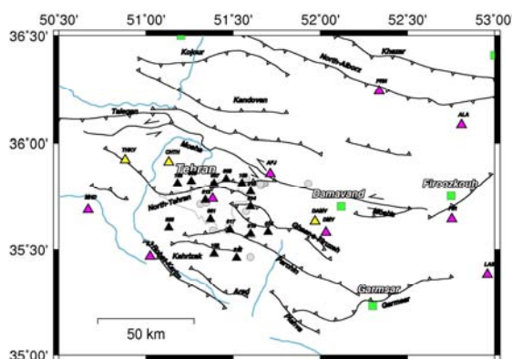
شکل (۸) - نقشه رومرکزهای رخدادهای منطقه تهران (3650-1a lon50-53) با گاف آزیموتی کمتر از ۲۷۰ درجه و خطای تعیین محل کمتر از ۲ کیلومتر برای طول و عرض جغرافیایی و ۵ کیلومتر برای عمق، شامل ۱۶ رخداد
