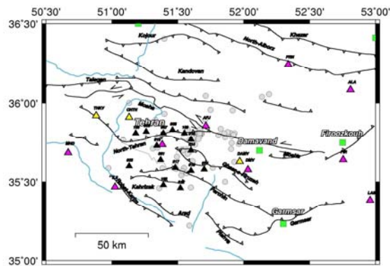
شکل (۶) - نقشه رومرکزهای رخدادهای منطقه تهران (3650-1a lon50-53) با گاف آزیموتی کمتر از ۲۷۰ درجه شامل ۷۴ رخداد
