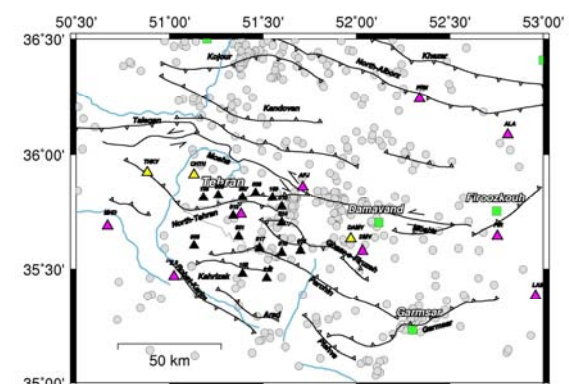
شکل (۵) - نقشه رومرکزهای تمام رخدادهای منطقه تهران (3650-1a lon50-53) شامل ۴۲۵ رخداد
