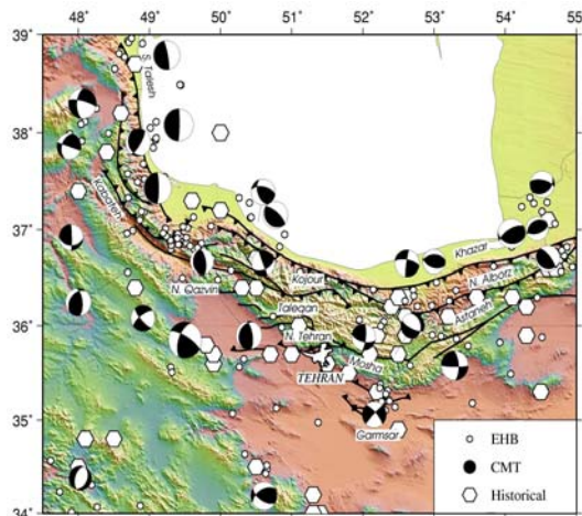
شکل (۱): نقشه تکتونیک ناحیه تهران و مجاورت آن. در شکل
