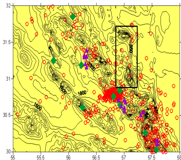
شکل ۵: نقشه لرزه زمین ساختی گسل لکرکوه در داخل کادر (دایره قرمز=زلزله دستگاهی زیر ۵ لوزی سبز= زلزله تاریخی و مثلث بنفش= زلزله دستگاهی بالای ۵)
