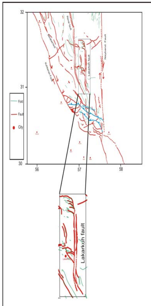
شکل ۳: نقشه ساختمانی منطقه مورد مطالعه و محدوده اطراف
