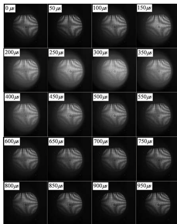
شکل ۳. روند زمانی تغییرات الگوی تداخلی مرکزی تداخل سنج حین عمل دمش نوری برای یک دیسک لیزر از لحظه تحریک لامپ های درخش تا ۱ میلی ثانیه پس از آن. ظرفیت خازن ۴۰۰ میکروفاراد و انرژی دمش ۱/۸ کیلوژول می باشد.
