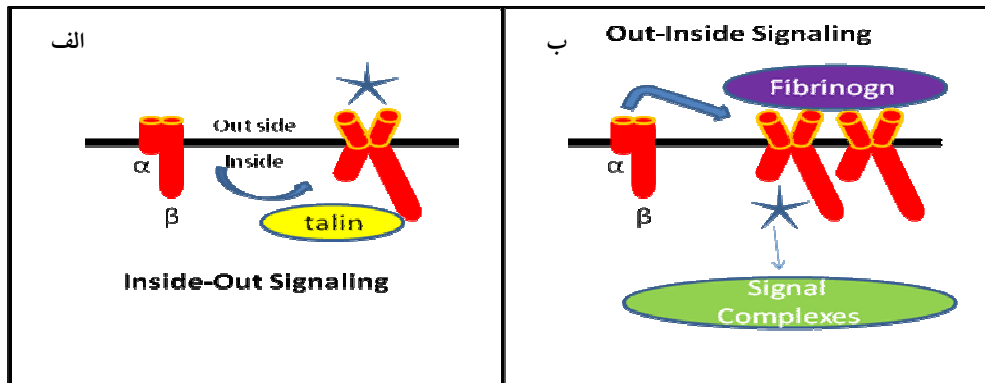
شکل ۱: انتقال پیام دوطرفه در اینتگرین‌ها الف: انتقال پیام از داخل سلول به خارج به داخل سلول
