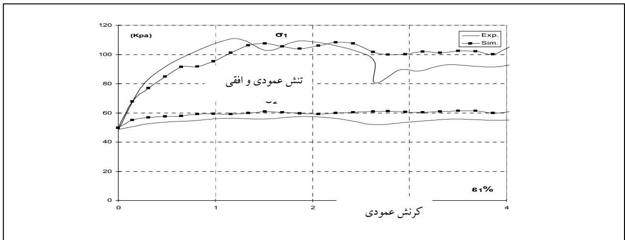
شکل ۲. تغییرات تنش‌های محوری و ثابت تابعی از کرنش محوری برای دو حالت عددی و تجربی
