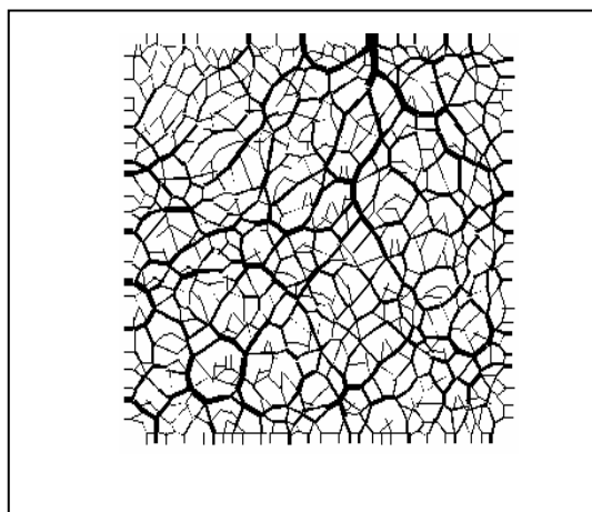
الف) \varepsilon_1 = 10\% (نیروی بیشینه ۱۶/۸ KN)
