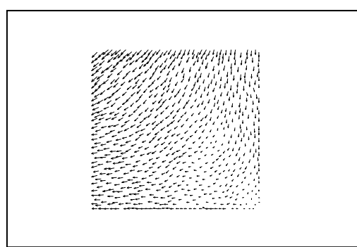
ب) تجربی (تغییر مکان بیشینه ۴۸/۹ میلیمتر)
