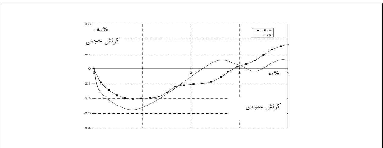
شکل ۳. تغییرات کرنش حجمی تابعی از کرنش محوری برای دو حالت عددی و تجربی
