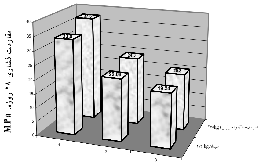
۵- ب) مخلوطهای حاوی ۲۷۰ کیلوگرم بر مترمربع مواد سیمانی
