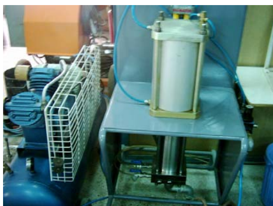
شکل ۴. تجهیزات آزمایش تعیین ضریب نفوذپذیری بتن
