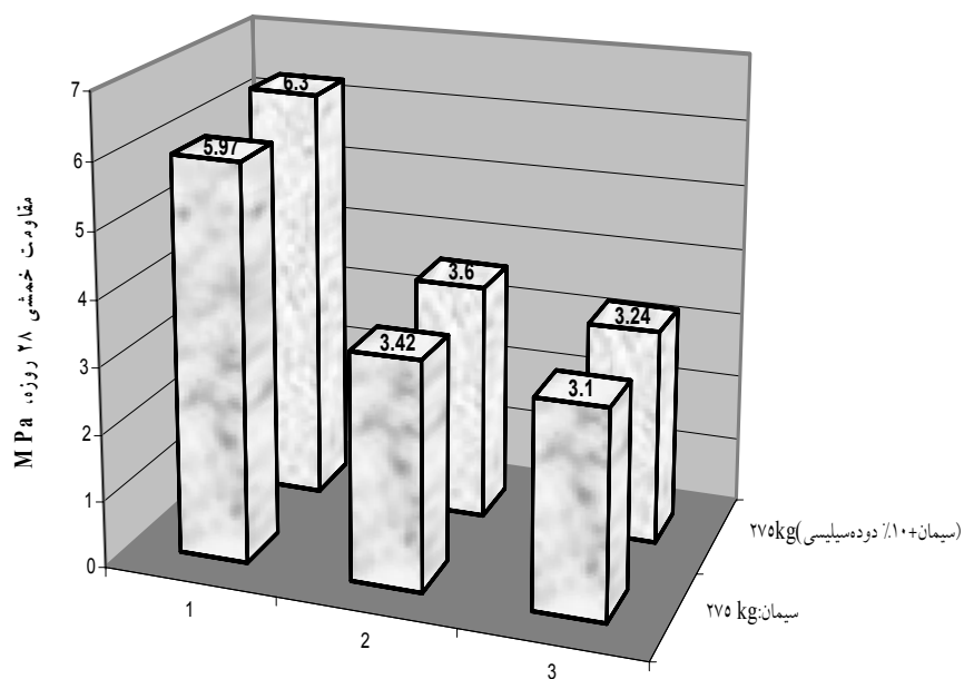
۶- ب) مخلوطهای حاوی ۲۷۵ کیلوگرم بر مترمربع مواد سیمانی
