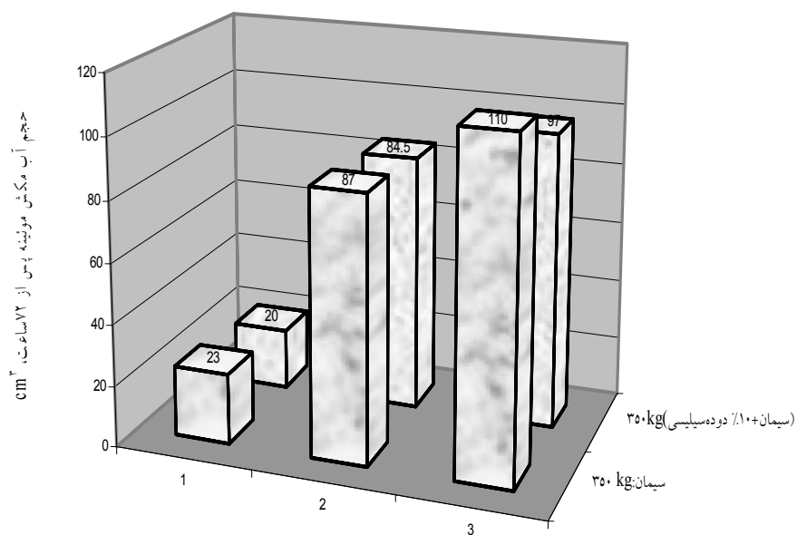
۷- ب) مخلوطهای حاوی ۲۷۵ کیلوگرم بر مترمربع مواد سیمانی
