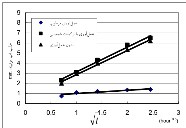
۹- ب) بتن غلتکی حاوی ۲۷۵ کیلوگرم سیمان و ۱۰ درصد دوده سیلیس
