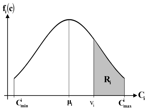
شکل ۱. تابع چگالی احتمالی ظرفیت کمان i و پارامترهای مربوط به محاسبه قابلیت اطمینان عملکرد آن
