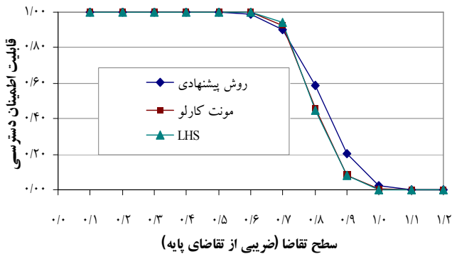
شکل ۴. مقایسه قابلیت اطمینان دسترسی زوج مبدأ - مقصد (او۵) از روش‌های مختلف
