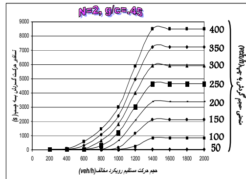
شکل ۱. منحنی‌های تأخیر گردش به چپ به ازای حجم‌های مختلف برای شرایط N=2, g/c=.45
