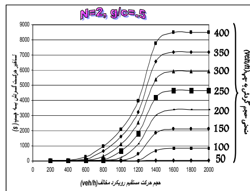
شکل ۳. منحنی‌های تأخیر گردش به چپ به ازای حجم‌های مختلف برای شرایط N=2, g/c=.5
