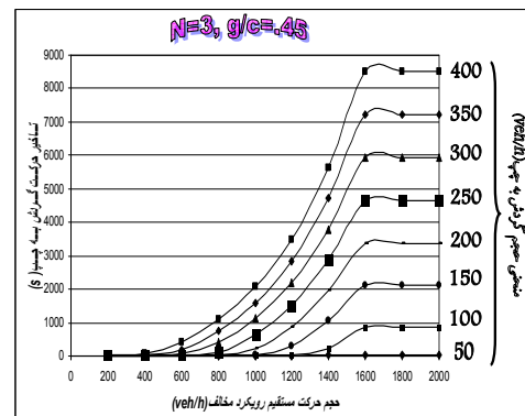
شکل ۲. منحنی‌های تأخیر گردش به چپ به ازای حجم‌های مختلف برای شرایط N=3, g/c=.45
