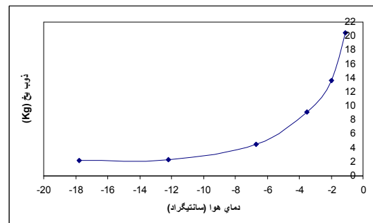
نمودار ۱. نشانگر نیاز استفاده از مقدار زیادتر نمک در درجه حرارت‌های پایین‌تر است [۱]
