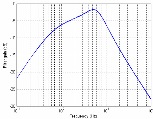
شکل ۲. دیاگرام بود (Bode) فیلتر استفاده شده برای وزن دادن
