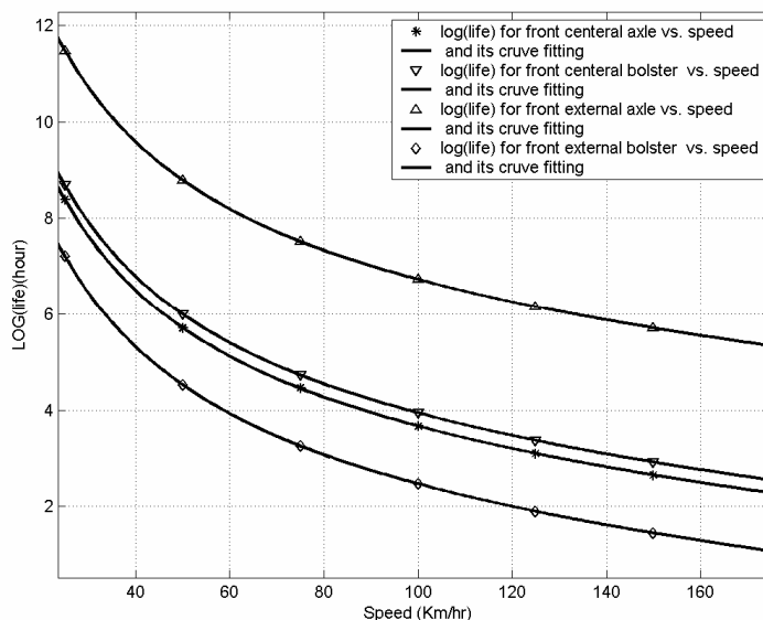
شکل ۱۱. نمودار عمر فنرهای جلو واگن در سرعت‌های مختلف برای نسبت \frac{e}{l} = 0.1 و ریل کلاس ۴
