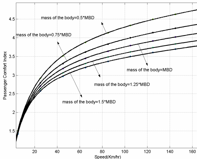
شکل ۱۰. نمودار مقابل تأثیر جرم واگن در راحتی سفر در نسبت \frac{e}{l} = 0.1 در وسط واگن در کلاس ریل ۴ نسبت به سرعت نشان می‌دهد.
